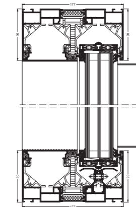
6 VERSIUNE 90/90 90/90 VERSION
