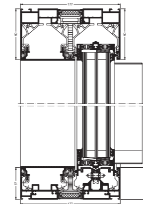
5 VERSIUNE 57/90 57/90 VERSION
